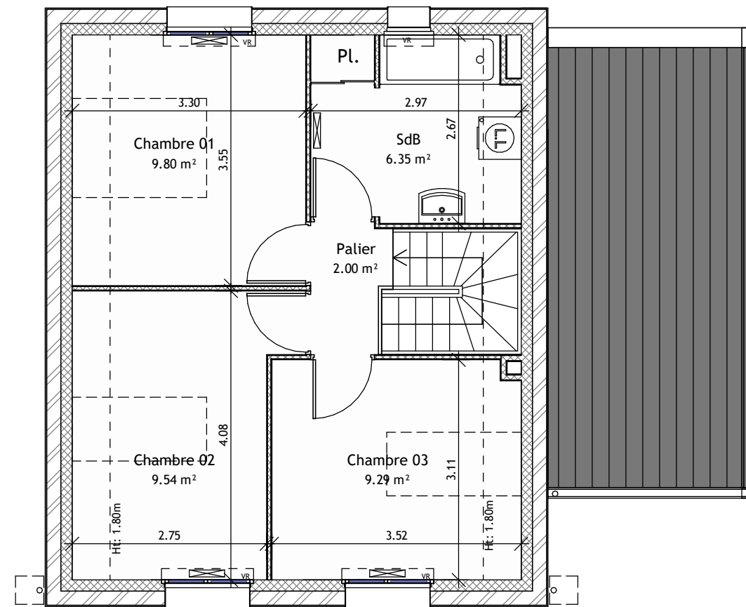
Etage 01 Ech : 1 : 75
