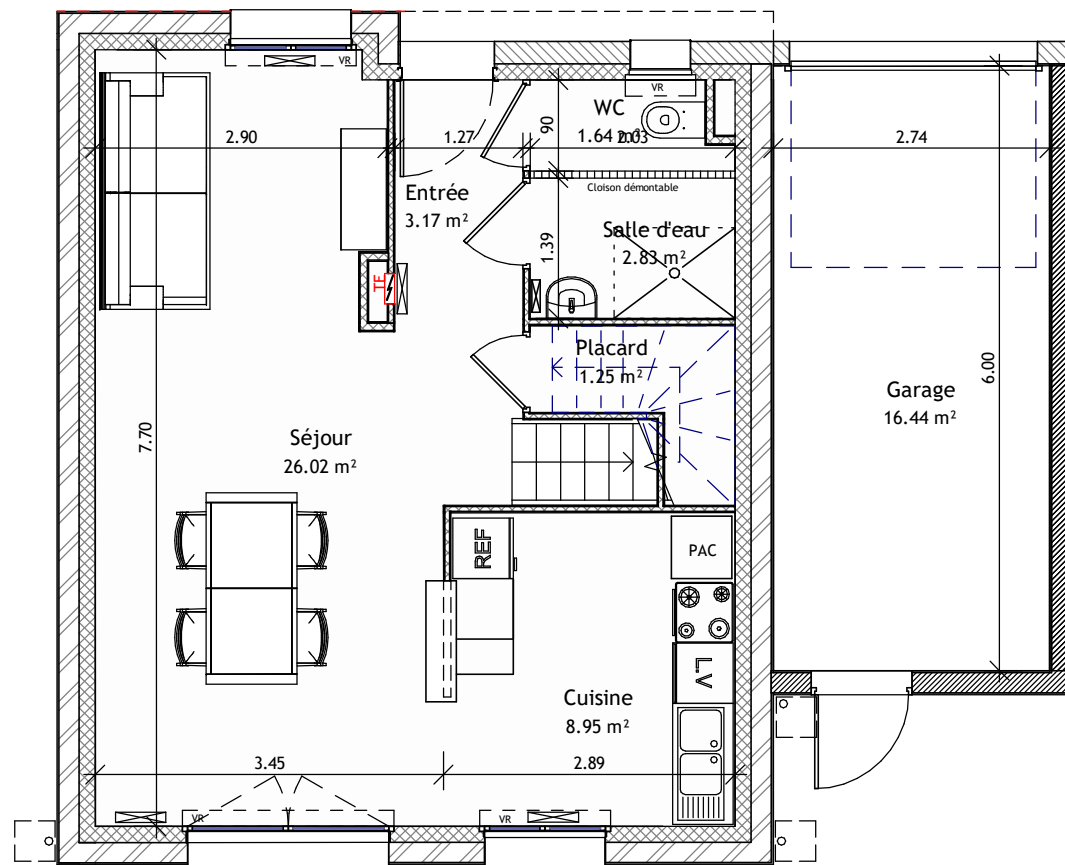
RDC Ech : 1 : 75
