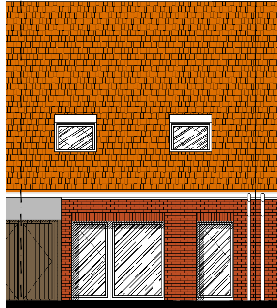
ELEVATION ARRIERE
