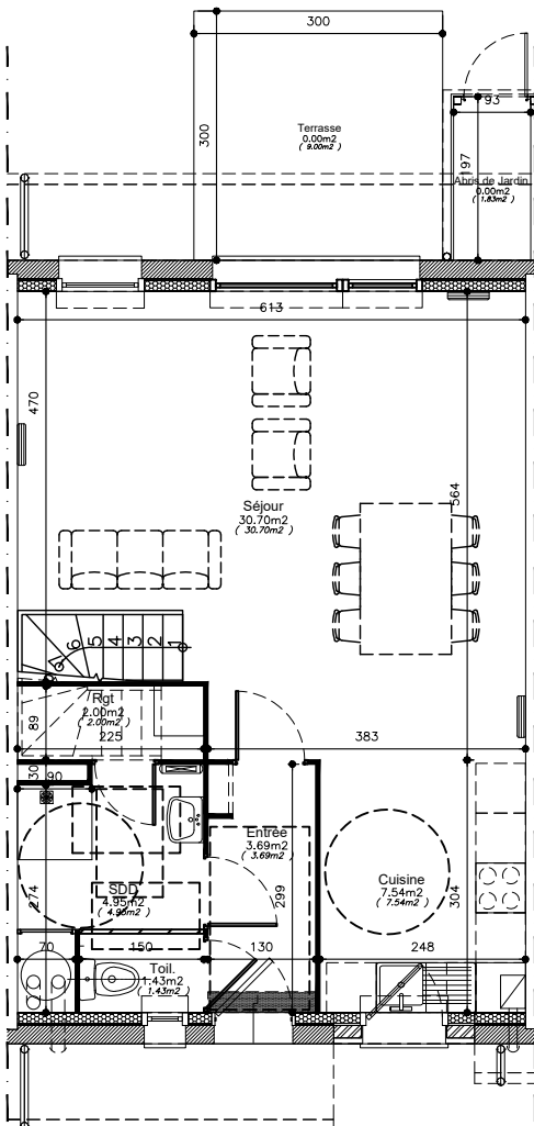
RDC
